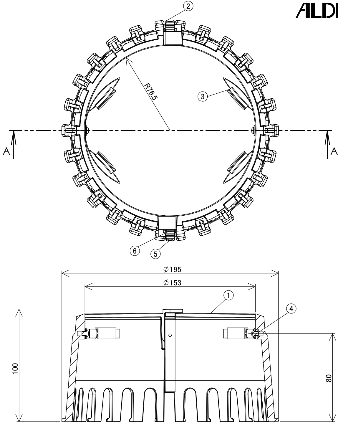
断面図 A-A
