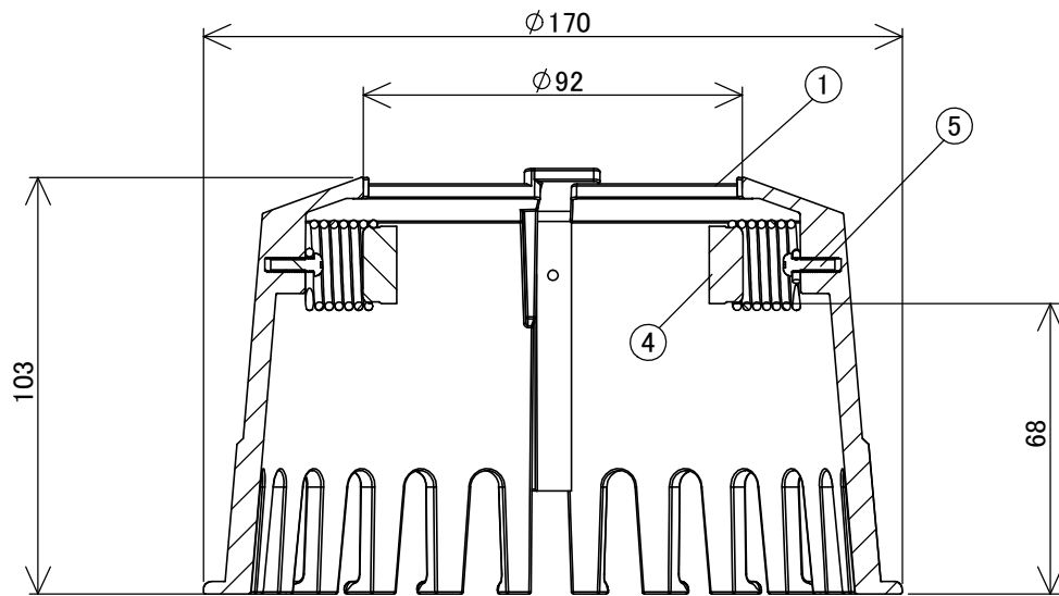
断面図 A-A
