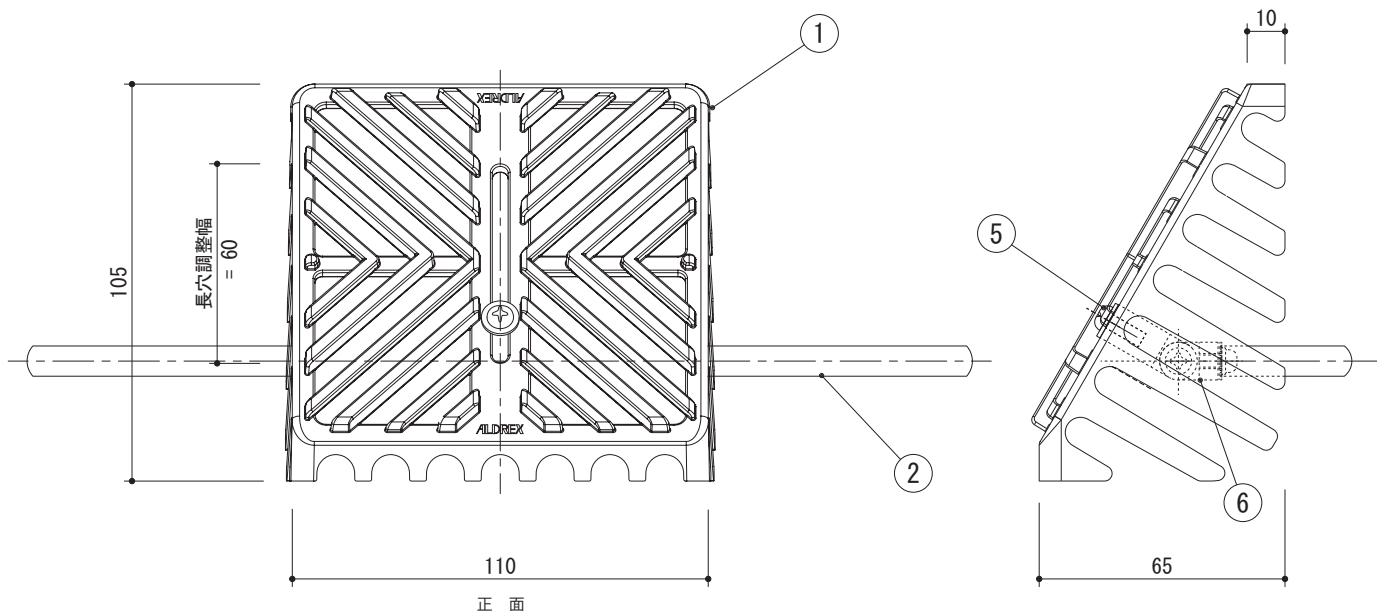
正面
